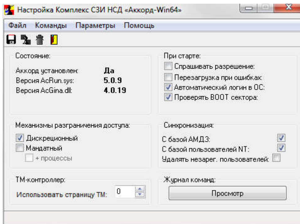
Рисунок 5 - Главное окно программы настройки комплекса «Аккорд»
